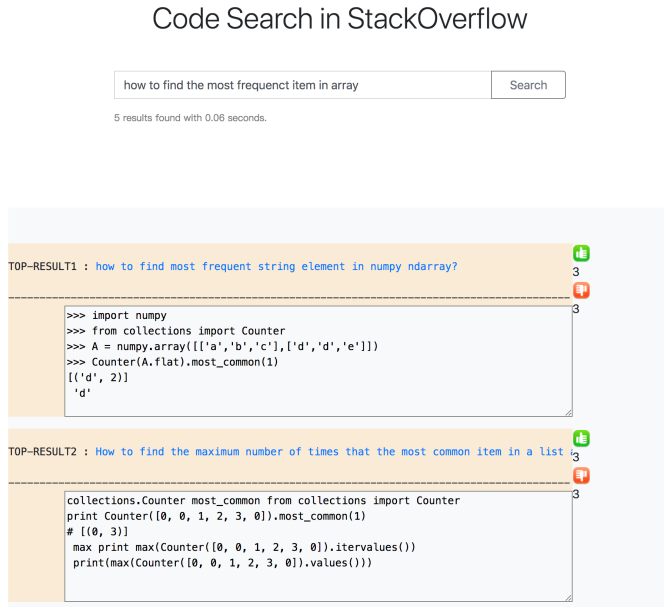
Fig. 12. Prototype of Que2Code
